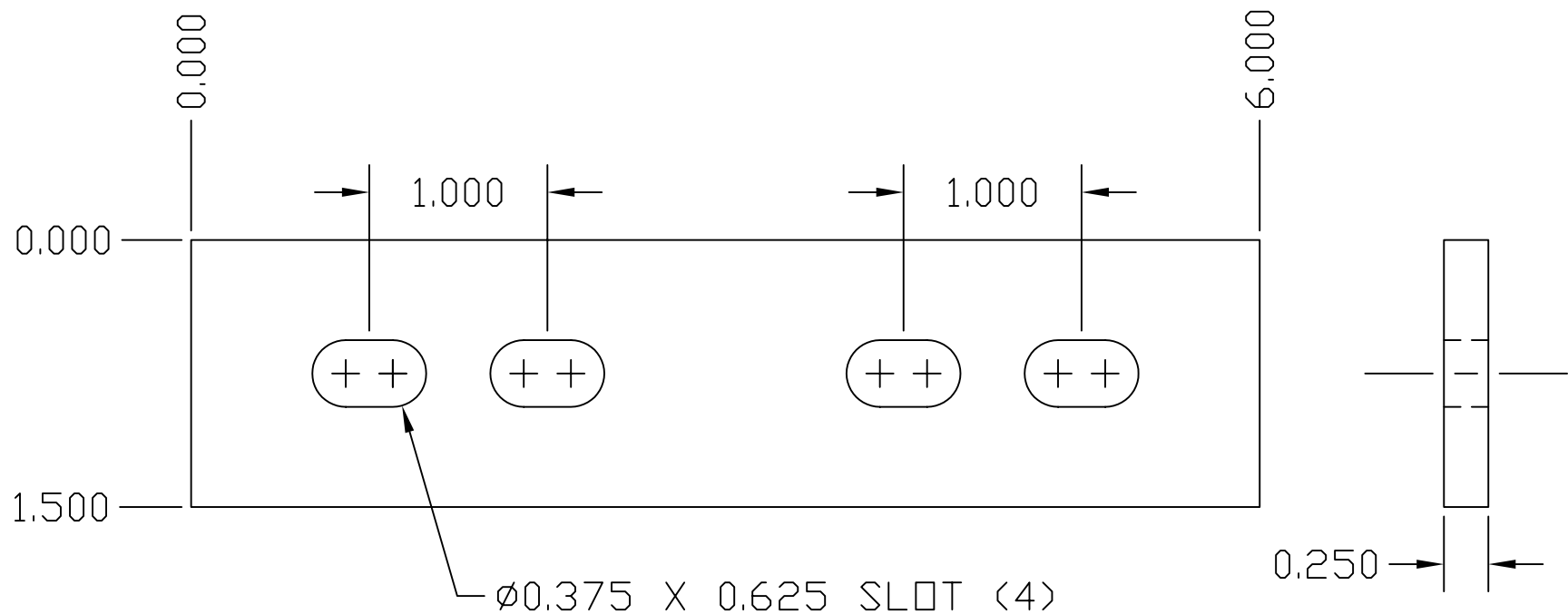
CU SPLICE PLATE
