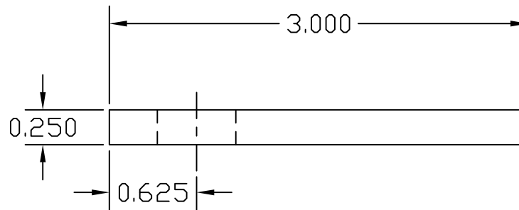
TINNED CU STRAIGHT 1-HOLE LUG
